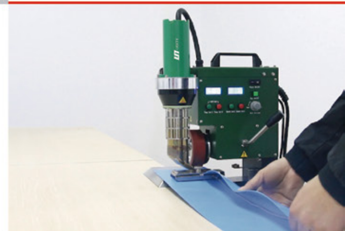
桌面式热风穿绳焊接 LST-PAU
