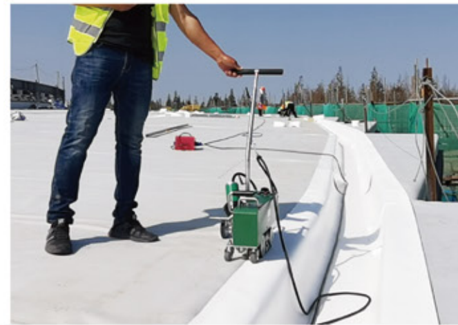
天沟边缘焊接 LST-WP4
