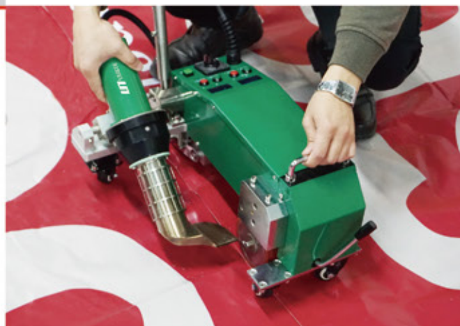
PVC 广告布的拼接 LST-MAT1
