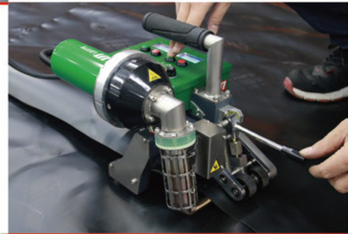
HDPE(1.2mm) 膜材焊接 LST700
