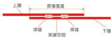
LST-GM1 焊接示意图
